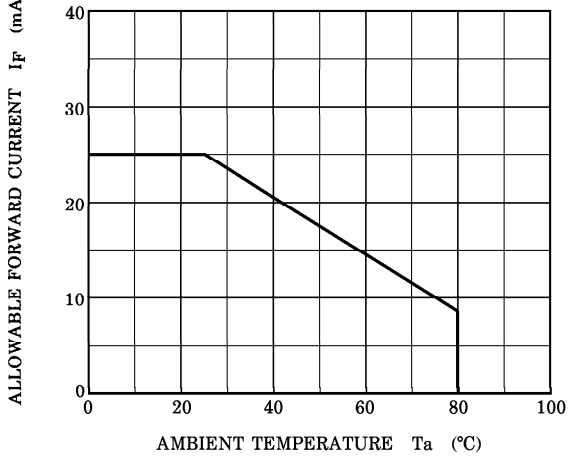
I_F - T_a
