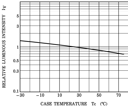
I_V - T_c
