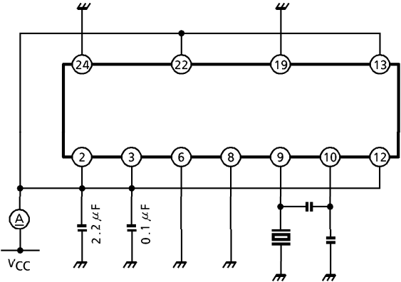
1. I_{CCO} , I_{CCS}
