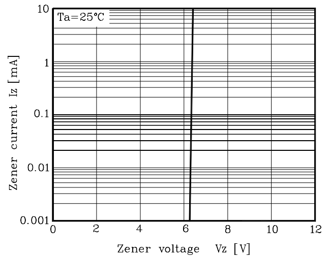
Fig. 2 I_Z - V_Z
