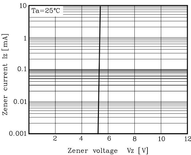
Fig. 2 I_Z - V_Z
