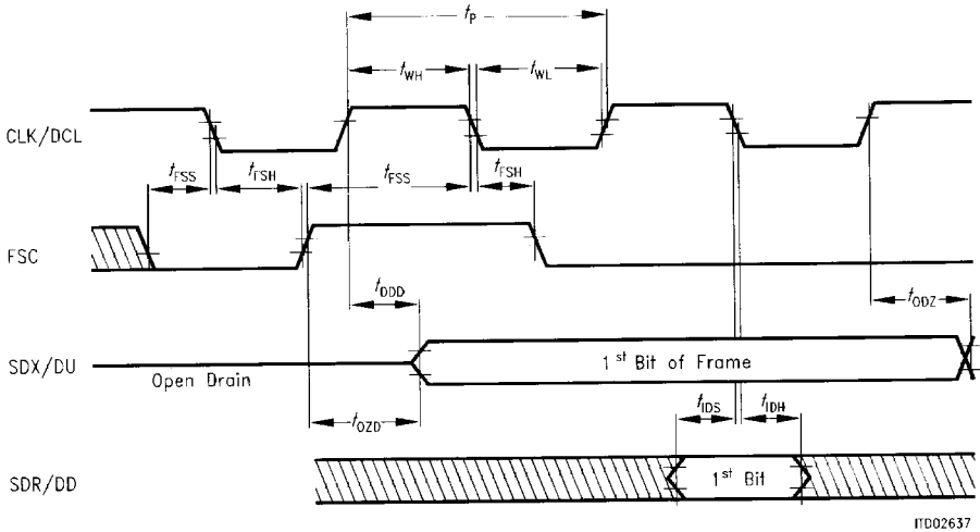
Figure 56 IOM ® -2 Interface Timing
