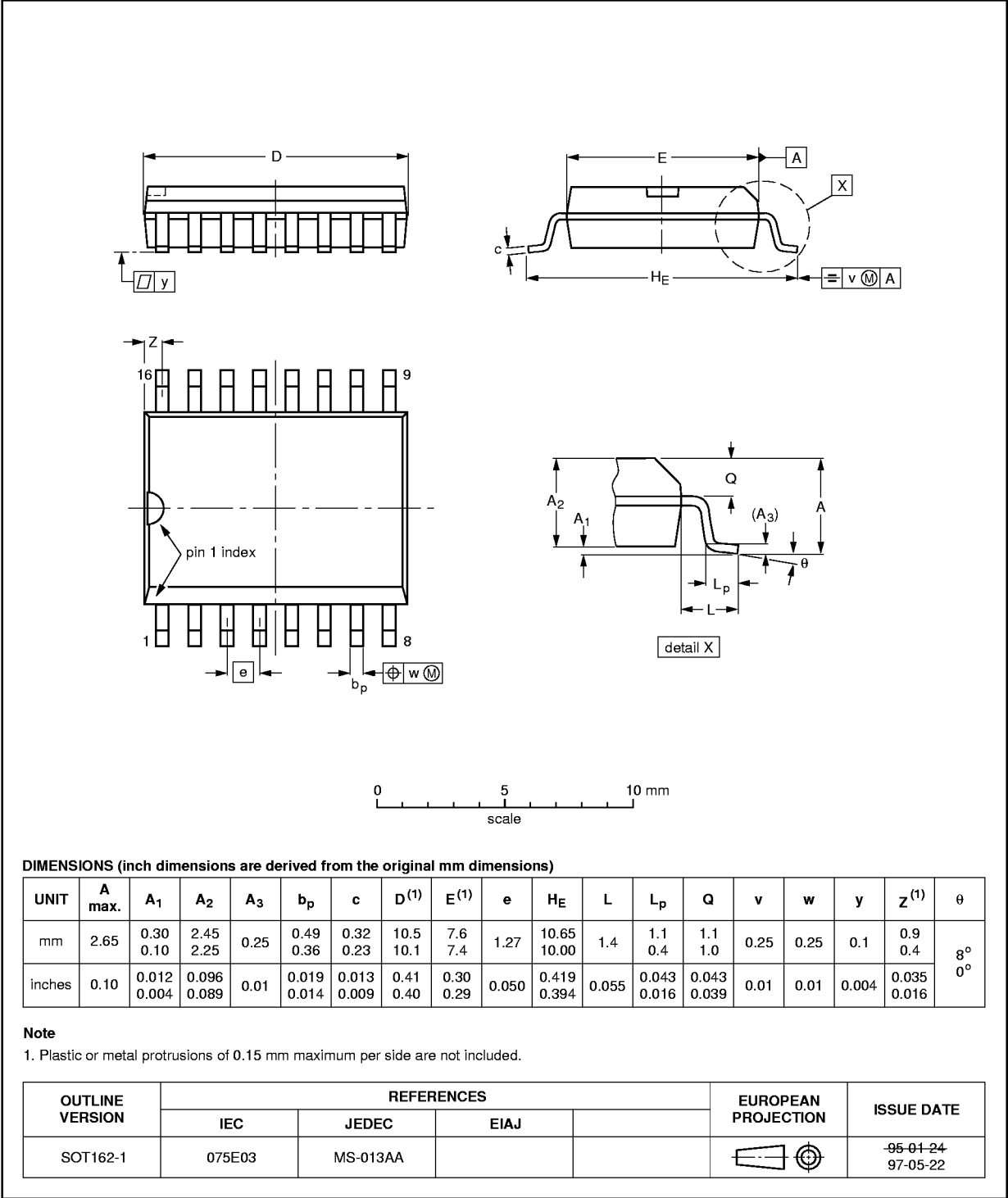
Fig 17. SOT162-1.
