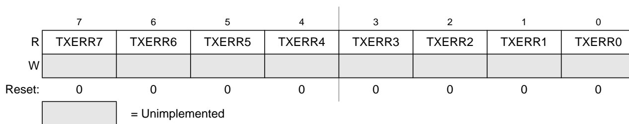
Figure 10-19. MSCAN Transmit Error Counter (CANTXERR)
