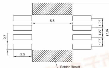
LAND PATTERNS(mm) 推奨ランド寸法
