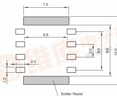
LAND PATTERNS(mm) 推奨ランド寸法
