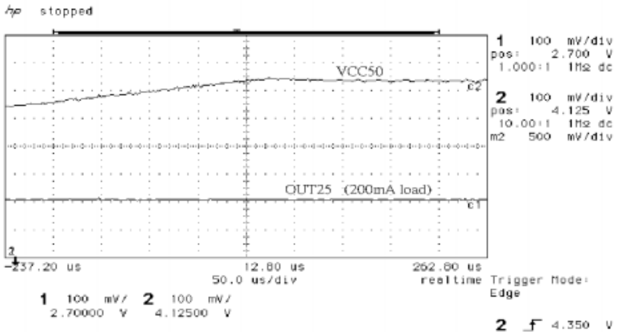
Fig. 6. 2.5V VCC50 Power Up (VSB50=5V)
