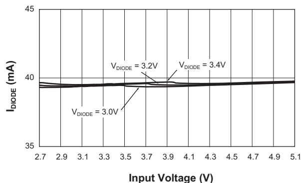
I_{DIODE} vs. Input Voltage (4x10mA)
