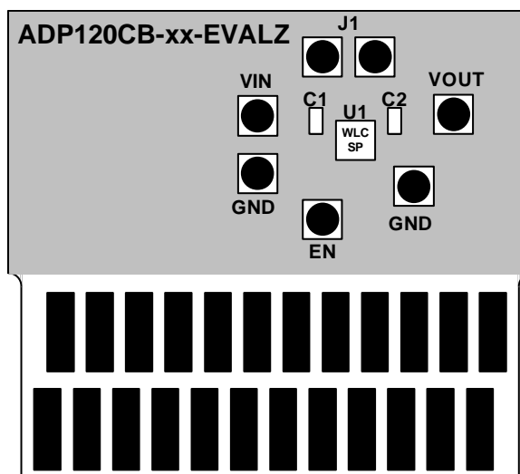
Figure 49. WLCSOP PCB Layout
