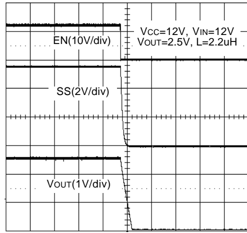
Shutdown (EN=GND)
