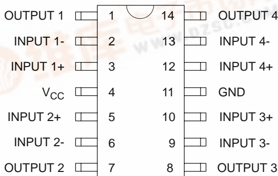
SOIC-14/DIP-14/TSSOP-14
