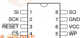
SOIC
