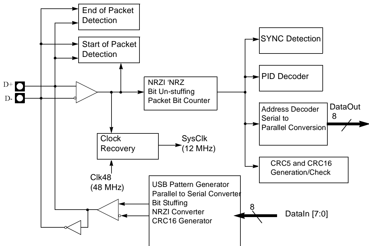
Figure 56. SIE Block Diagram
