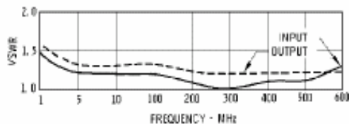
VSWR
