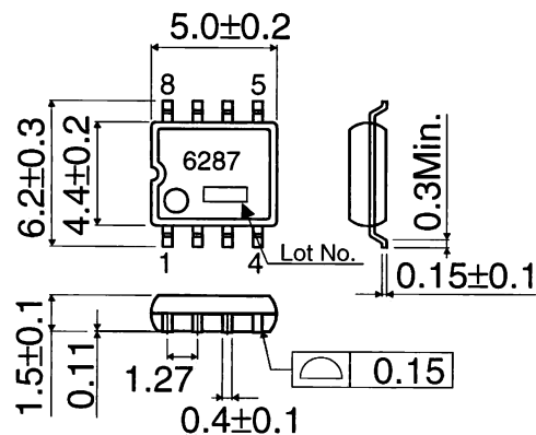
SOP8 (Unit:mm)
