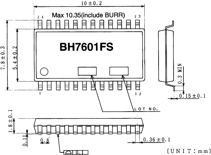
PKG : SSOP-A24
