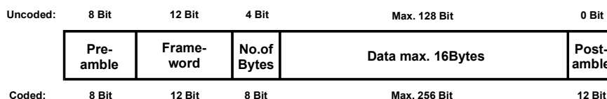
Fig. 10: Dataformat
