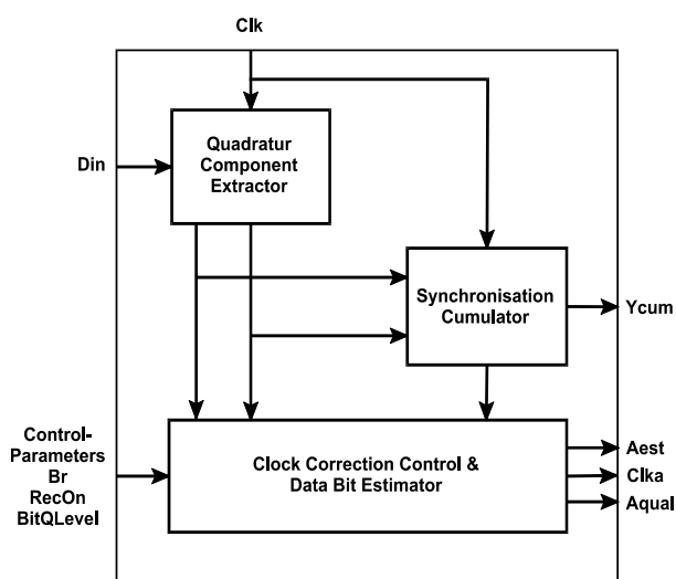
Fig. 3: Bit Estimator
