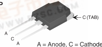
TO-3 P
