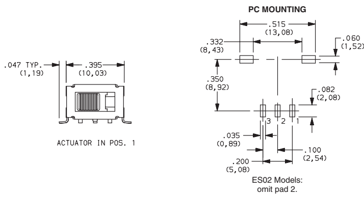
ES01MSABE Horizontal Actuation SPDT
