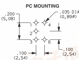
ES02 Models: omit hole 2.
