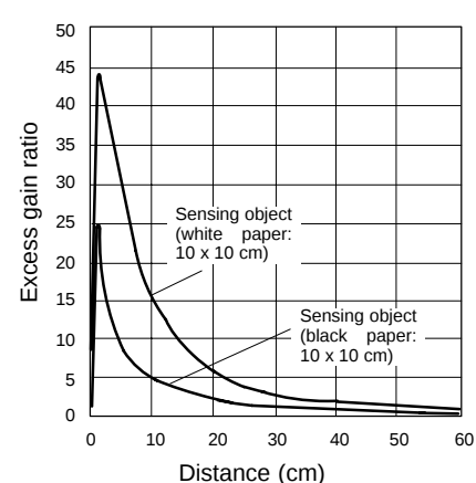
E3F2-DS30□4 E3F2-DS30□4-P1
