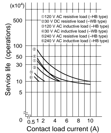
Life curve (10 A type, breake side (N.C.))
