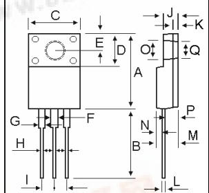
ITO-220AB
