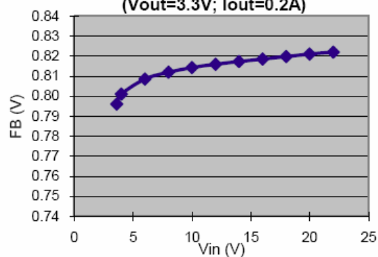
FSP3131 Vin vs. FB (Vout=3.3V; Iout=0.2A)
