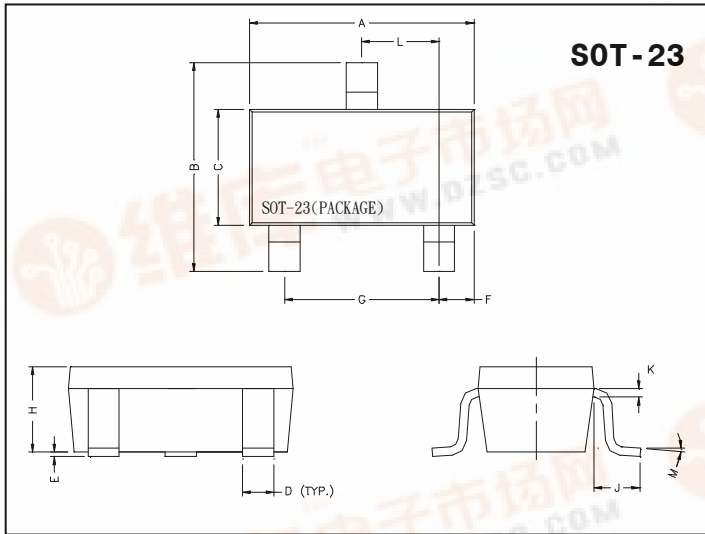
Style : Pin1. Anode 2. Anode 3. Cathode
