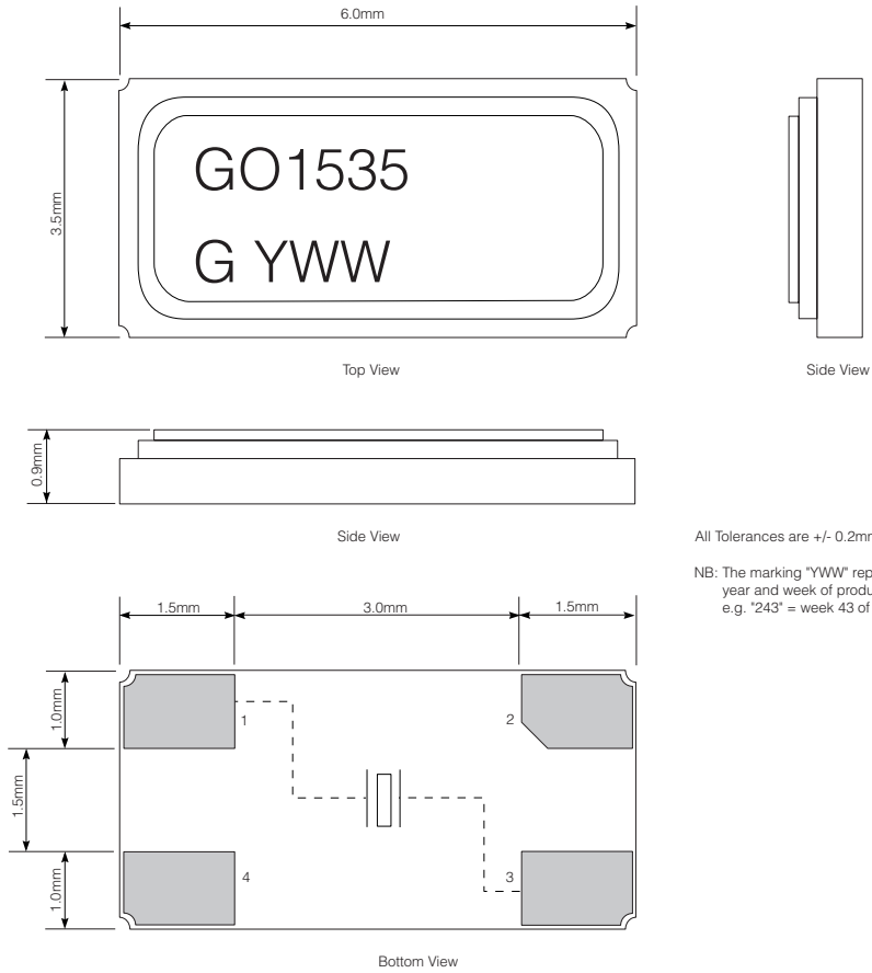
Fig. 2 Package Dimensions
