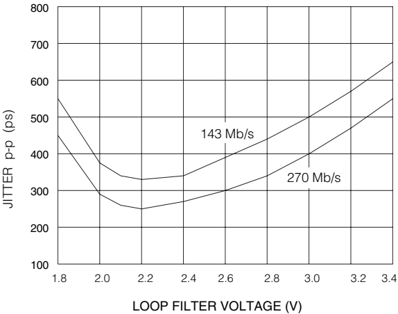
Fig. 16 Output Jitter
