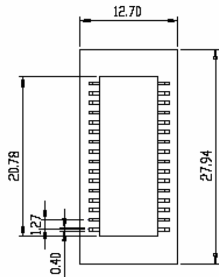
HCTL-2021 SHOWN
