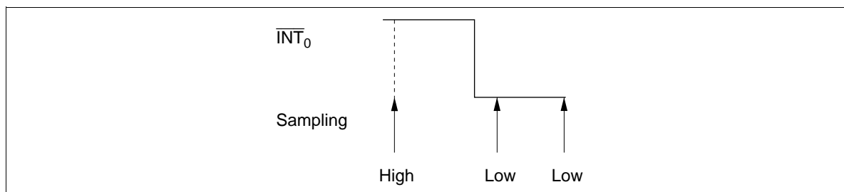
Figure 20 Edge Detection
