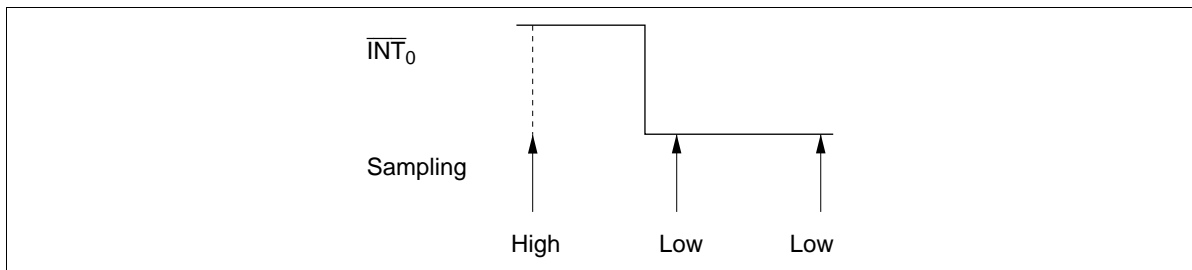
Figure 23 Edge Detection
