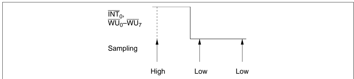
Figure 23 Edge Detection
