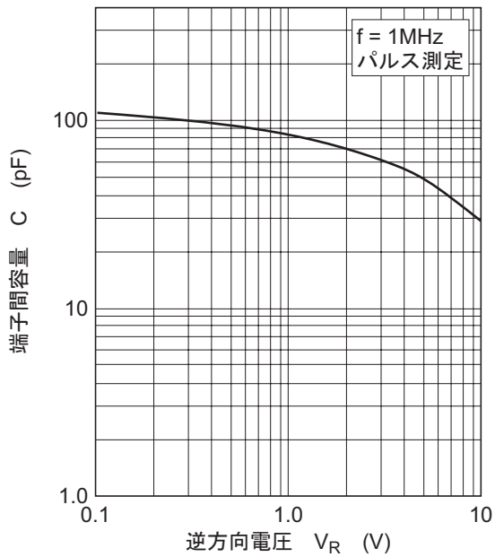
図3. 端子間容量 対 逆方向電圧
