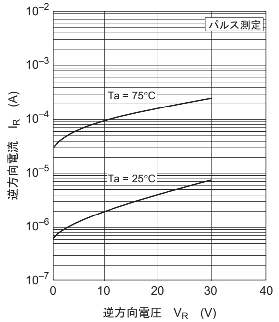
図2. 逆方向特性
