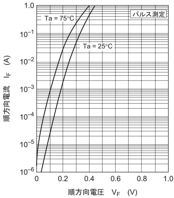
図1. 順方向特性
