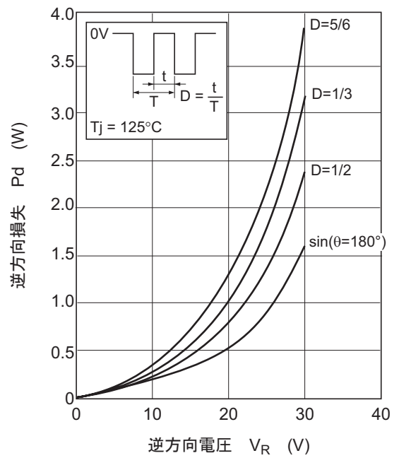
图5. 逆方向损失 对 逆电压特性
