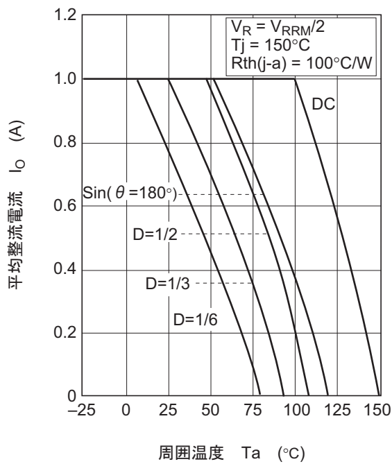
图6. 平均整流电流 对 周围温度特性
