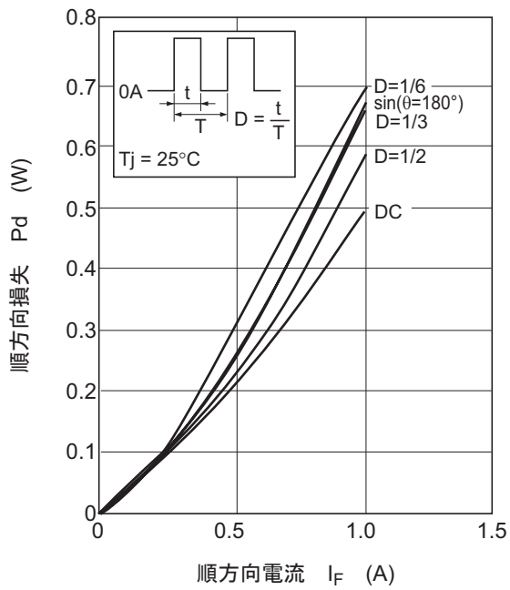
图4. 顺方向损失 对 顺电流特性
