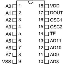
HT12E -18 DIP-A
