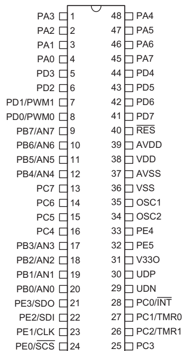
HT46RB50 – 48 SSOP-A
