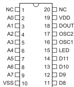
HT6014 -20 SOP-A
