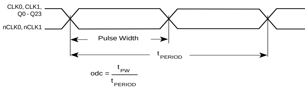
FIGURE 7 - odc & t_{PERIOD}
