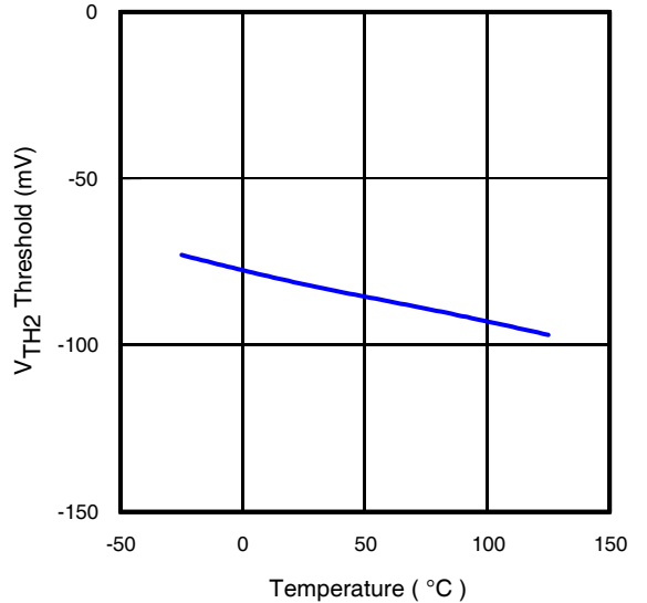
Fig 4. V TH2 vs. Temp.
