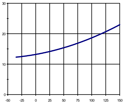
Figure 11 - Rds(on) (mΩ) vs Tj (°C)
