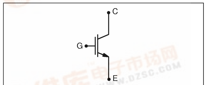
Fig.2 ITH08F06 circuit
