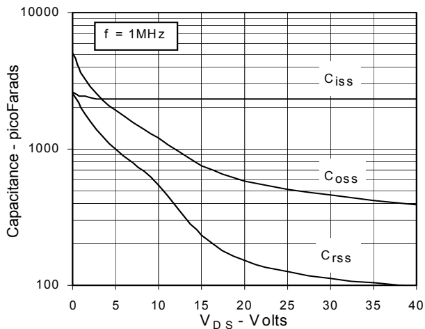
Fig. 11. Capacitance
