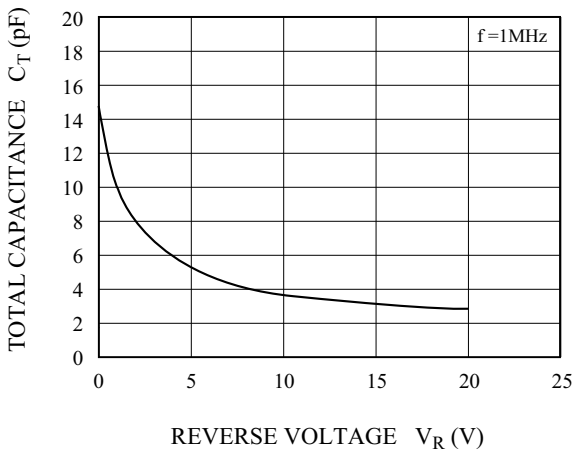
C_T - V_R
