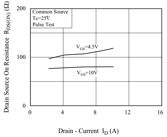
Fig2. R_{DS}-I_D
