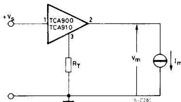
Fig. 1 - Test circuit.
