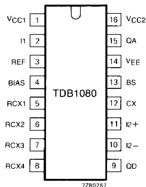
Fig. 2 Pinning diagram.
