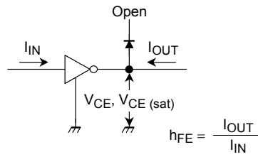
2. V_{CE(sat)} , h_{FE}
