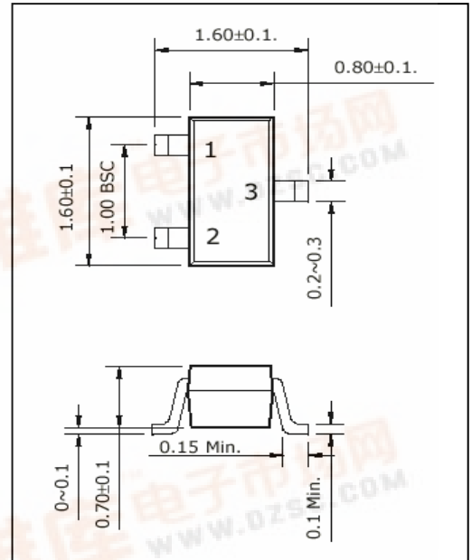
SOT 523
