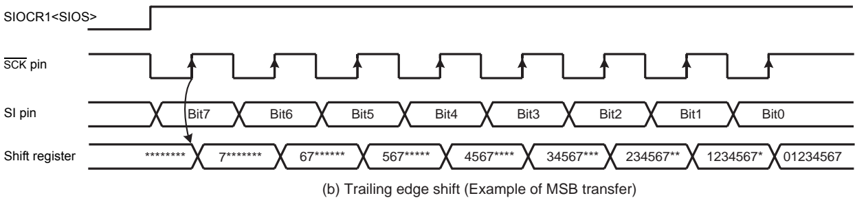
Figure 9-4 Shift Edge
