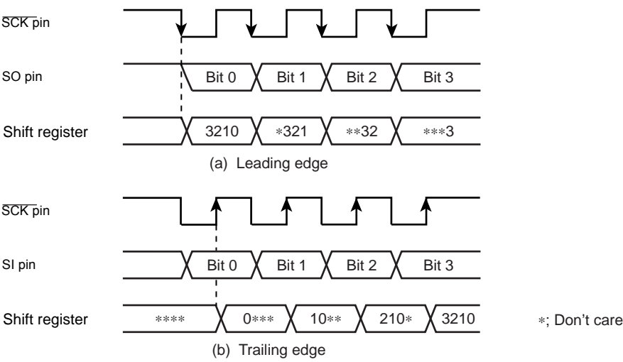
Figure 11-5 Shift edge
