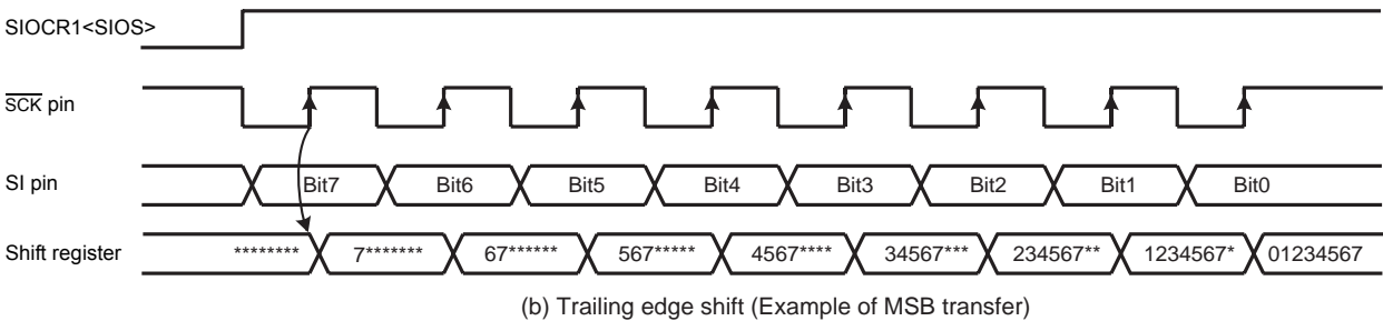
Figure 11-4 Shift Edge
